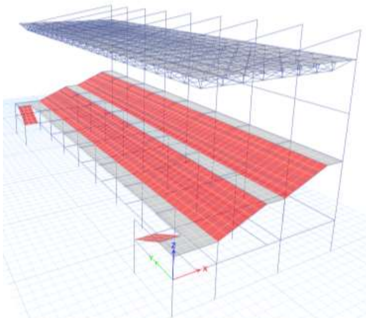
Μοντέλο ETABS κερκίδων σταδίου
