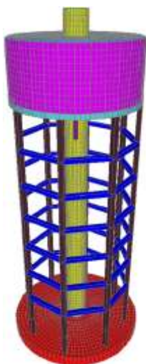
Στατικό προσομοίωμα υδατόπυργου χωρητικότητας 500\text{m}^3 νερού
